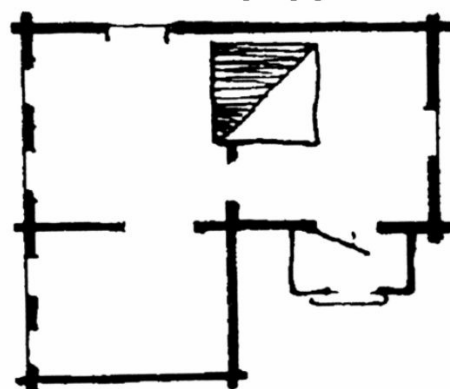
Связь (изба + сени). Клеть с перерубом
