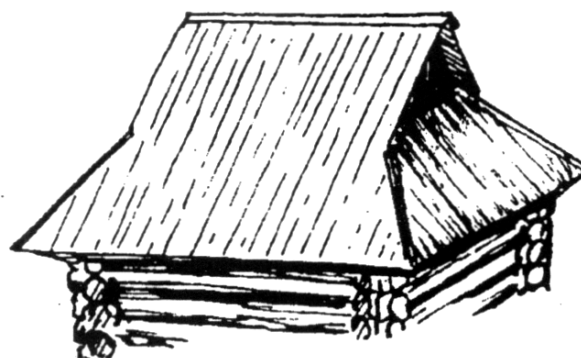
Крыша с козырьком
